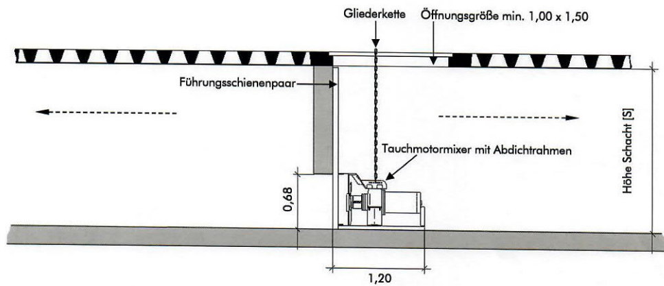
Schnitt schematisch
