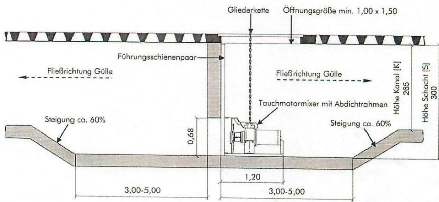
Schnitt schematisch
